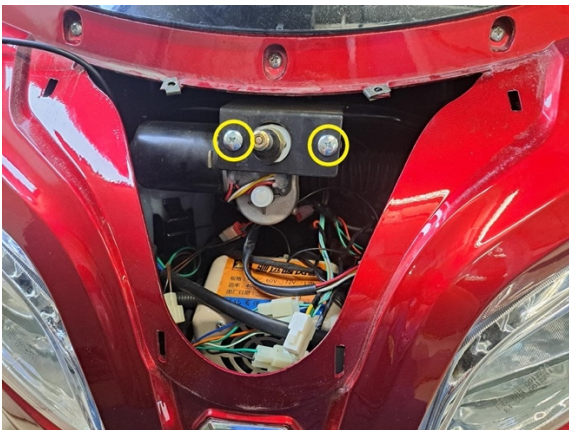
Irrota tuulilasipyyhkijän moottorin kiinnitysruuvit, (ristipäämeisseli ph2) joilla on vastamutteri. (kiintoavain 10 mm).
